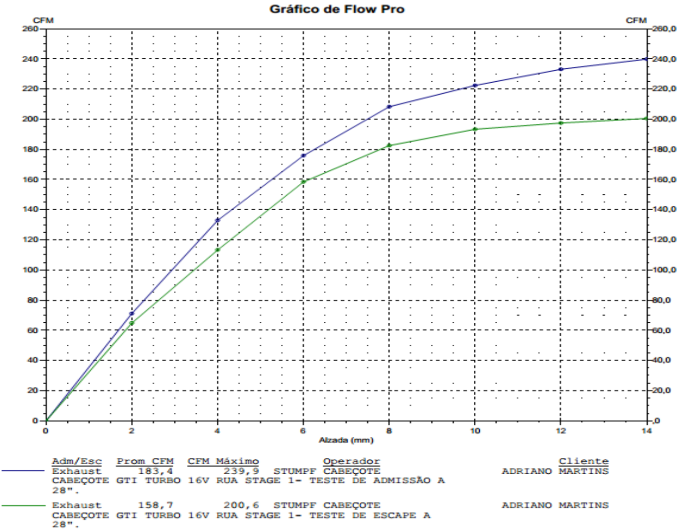
GRAFICO DE FLUXO- CABEÇOTE GTI TURBO 16V RUA STAGE 1- ADRIANO MARTINS
