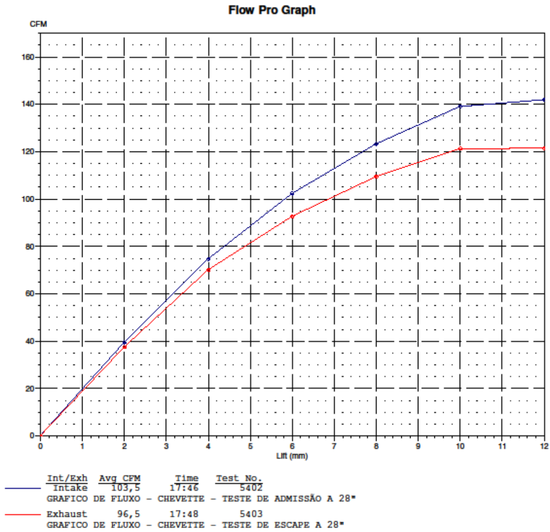
GRAFICO DE FLUXO - CHEVETTE - TESTE DE ADMISSÃO E ESCAPE A 28"
