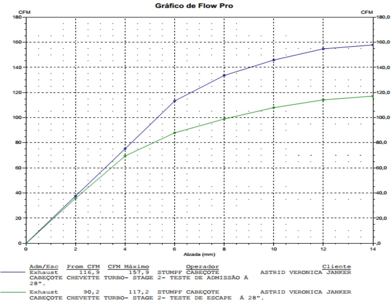
GRAFICO DE FLUXO-CABEÇOTE CHEVETTE TURBO- STAGE 2- ASTRID VERONICA JANKER
