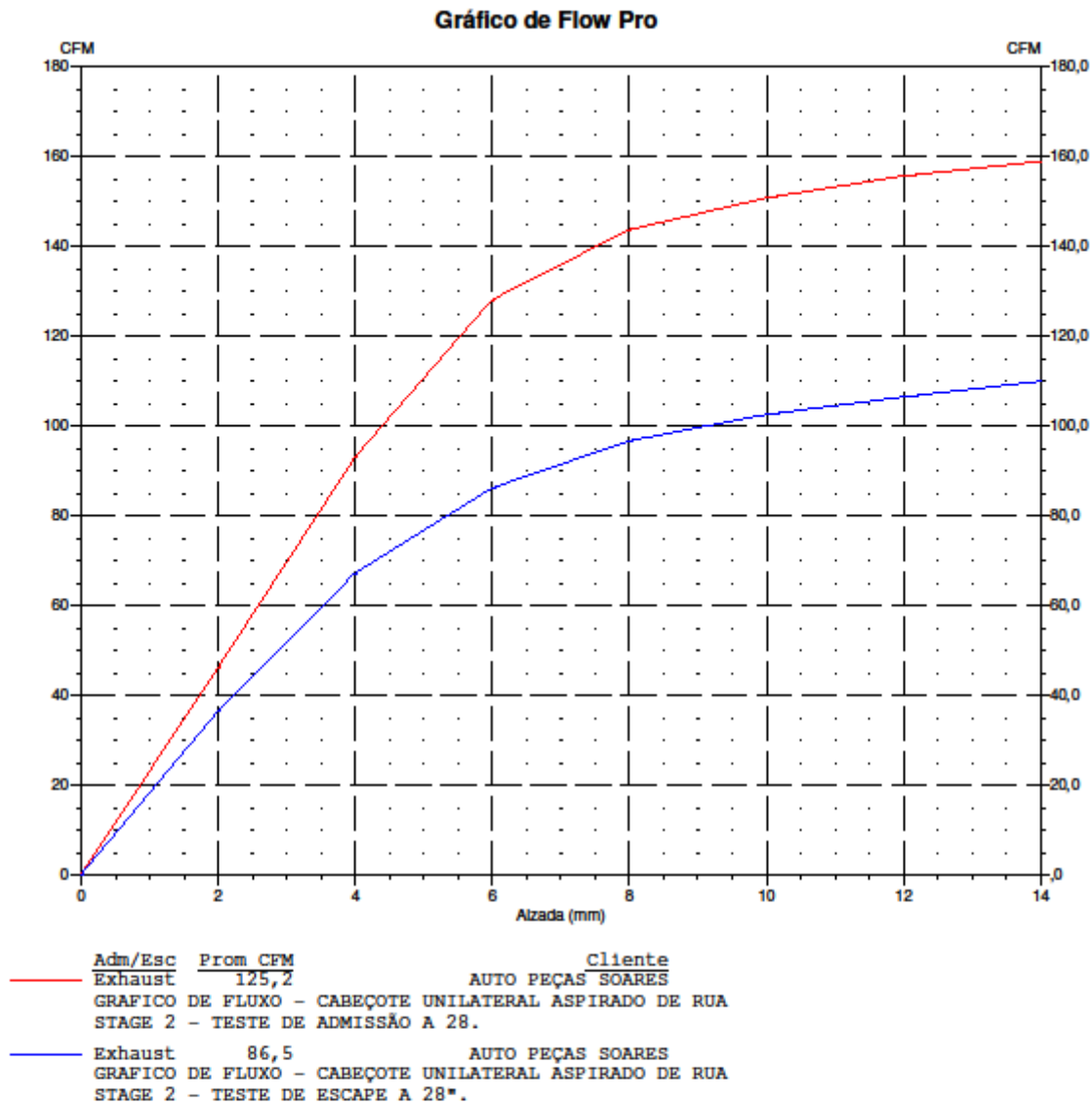
GRAFICO DE FLUXO - CABEÇOTE UNILATERAL ASPIRADO DE RUA STAGE 2 - AUTO PEÇAS SOARES
