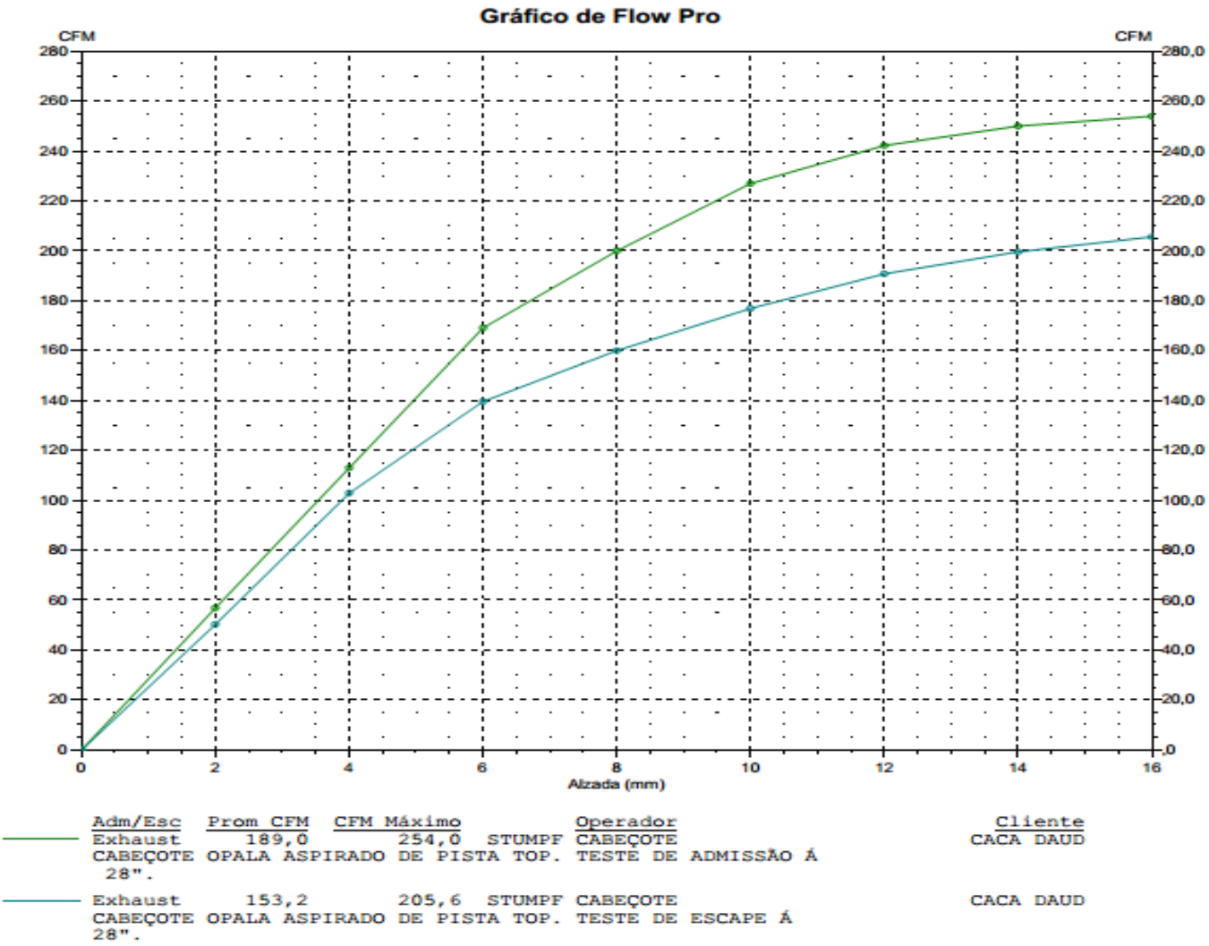
GRAFICO DE FLUXO- CABEÇOTE OPALA ASPIRADO DE PISTA TOP. CACA DAUD
