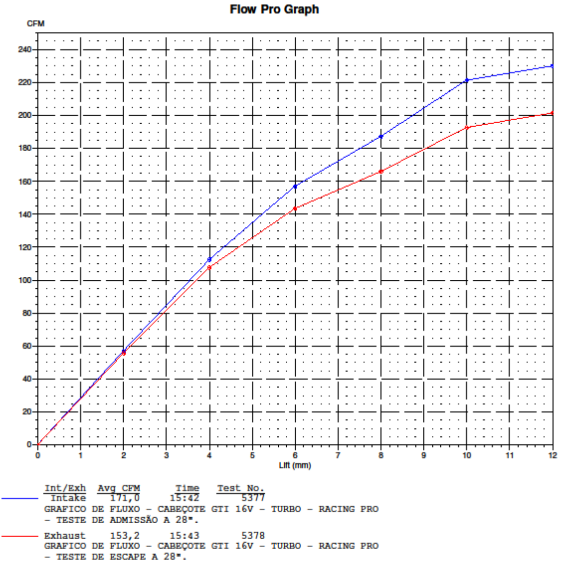
GRAFICO DE FLUXO - CABEÇOTE GTI 16V - TURBO - RACING PRO - TESTE DE ADMISSÃO E ESCAPE A 28"
