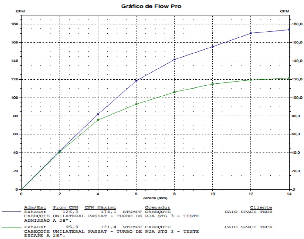
GRAFICO DE FLUXO - CABEÇOTE UNILATERAL PASSAT - TURBO DE RUA STG 3 - CAIO TAVARES DA SILVA.
