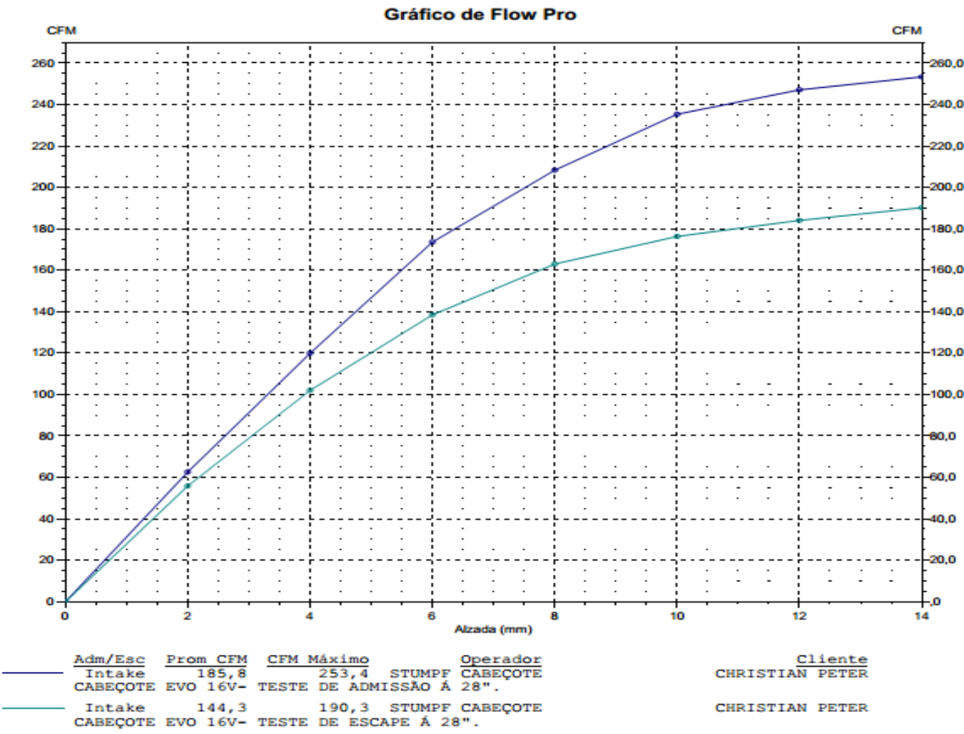
GRAFICO DE FLUXO-CABEÇOTE EVO 16V- CRISTIAN PETER
