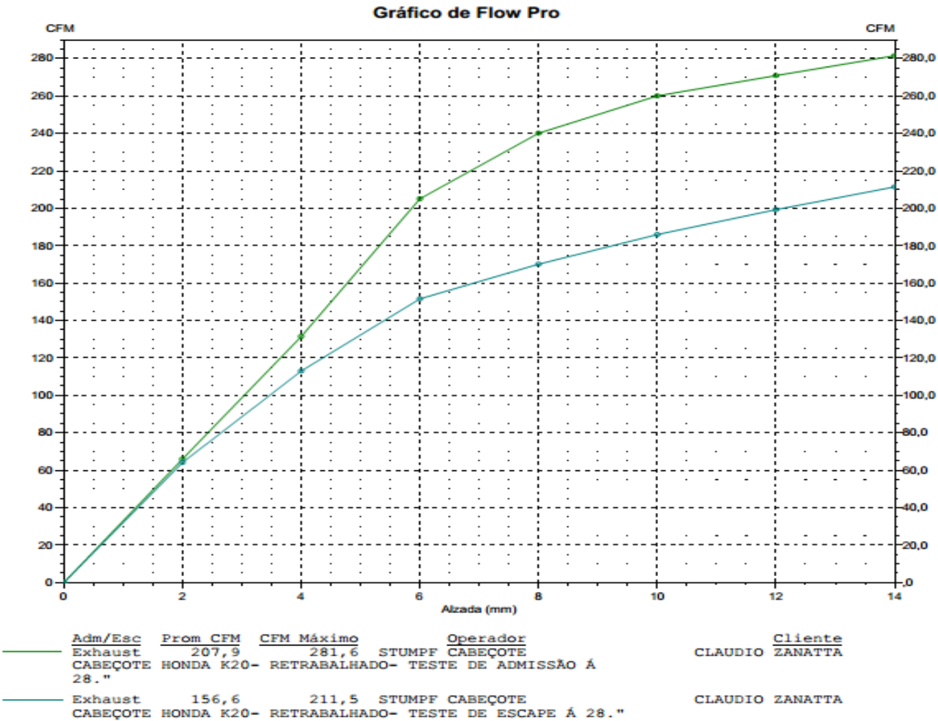
GRAFICO DE FLUXO-CABEÇOTE HONDA K20- RETRABALHADO- CLAUDIO ZANATTA
