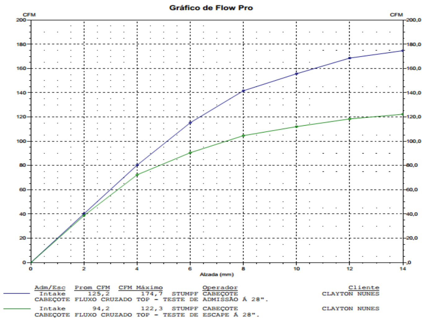
GRAFICO DE FLUXO-CABEÇOTE FLUXO CRUZADO TOP - CLAYTON DA SILVA NUNES
