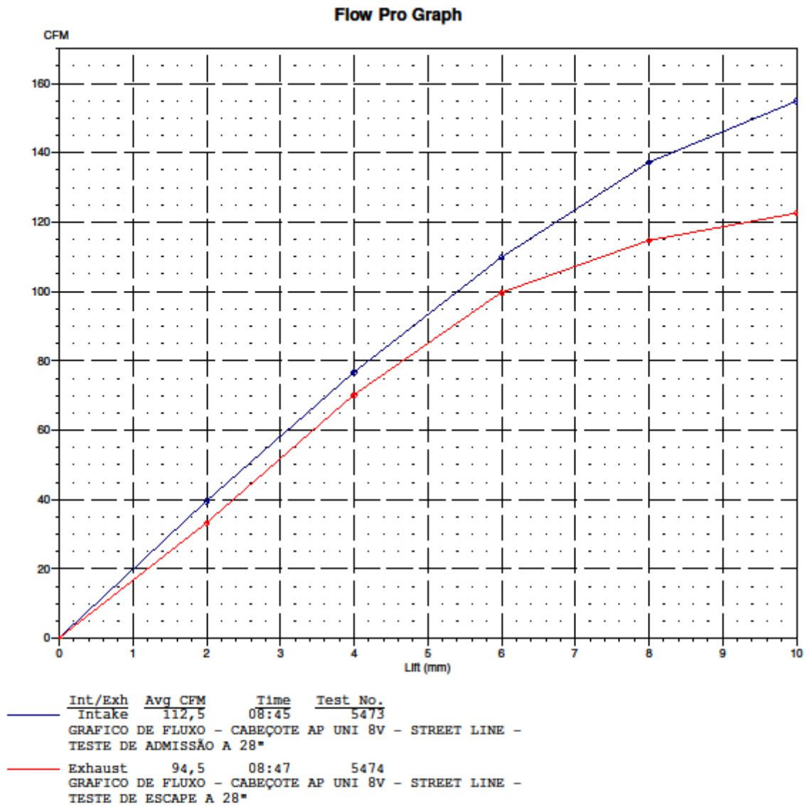
GRAFICO DE FLUXO - CABEÇOTE AP 8V UNI - STREET LINE - TESTE DE ADMISSÃO E ESCAPE A 28"
