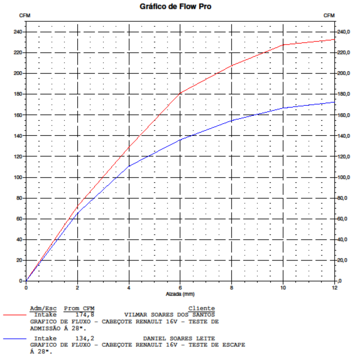
GRAFICO DE FLUXO - CABEÇOTE RENAULT 16V - DANIEL SOARES LEITE.
