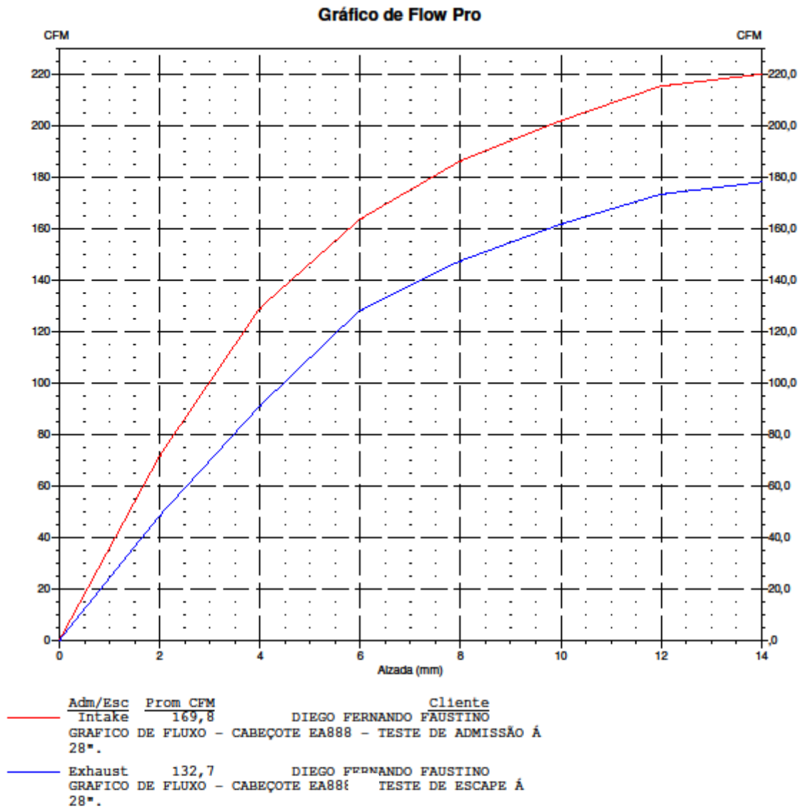
GRAFICO DE FLUXO - CABEÇOTE EA888 - DIEGO FERNANDO FAUSTINO.
