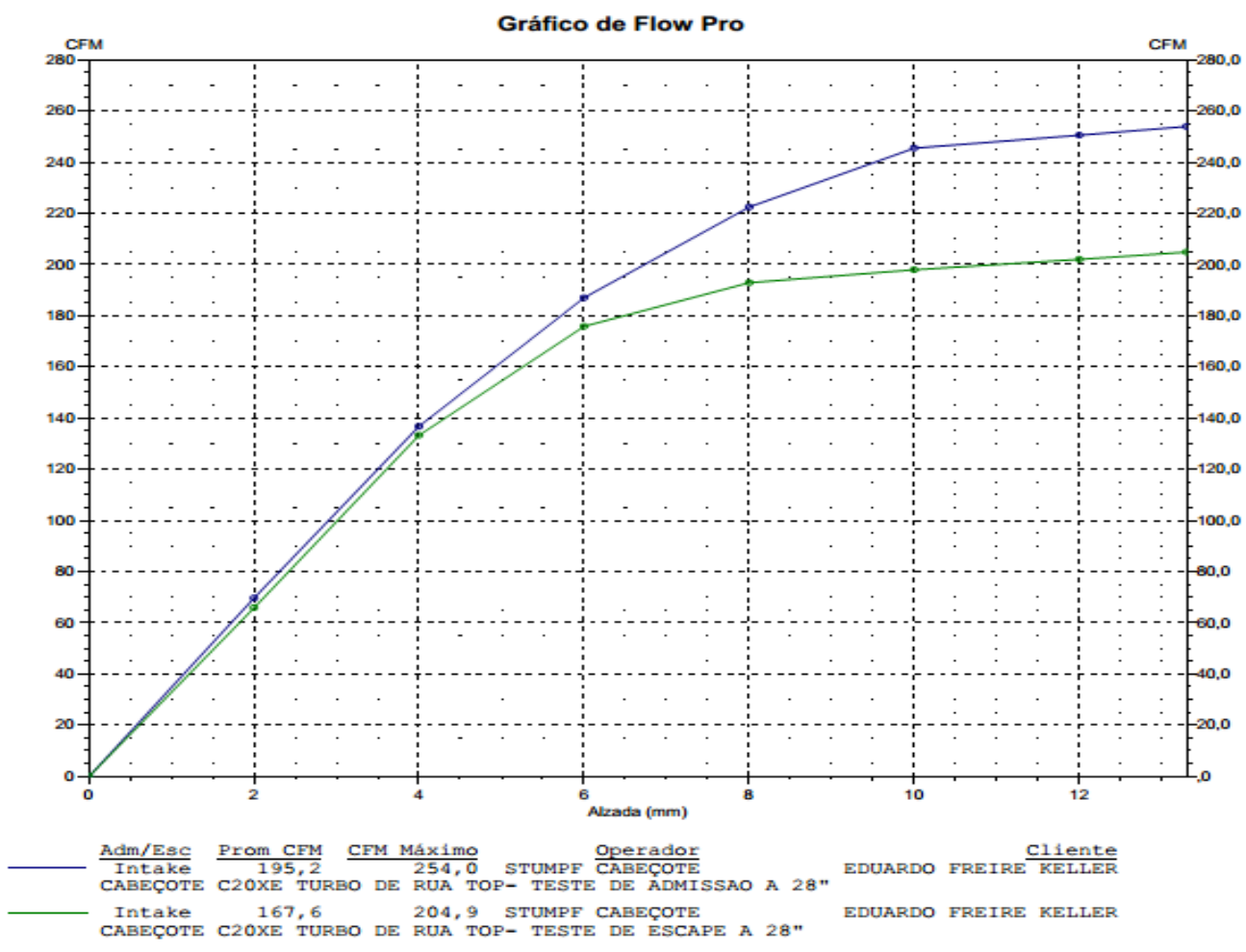
GRAFICO DE FLUXO - CABEÇOTE C20XE TURBO DE RUA TOP- EDUARDO FREIRE KELLER.
