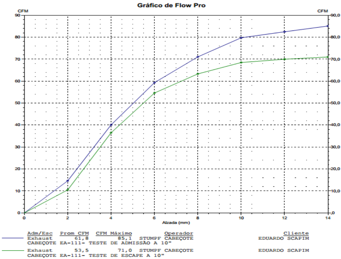
GRAFICO DE FLUXO -CABEÇOTE EA-111- EDUARDO SCAPIM
