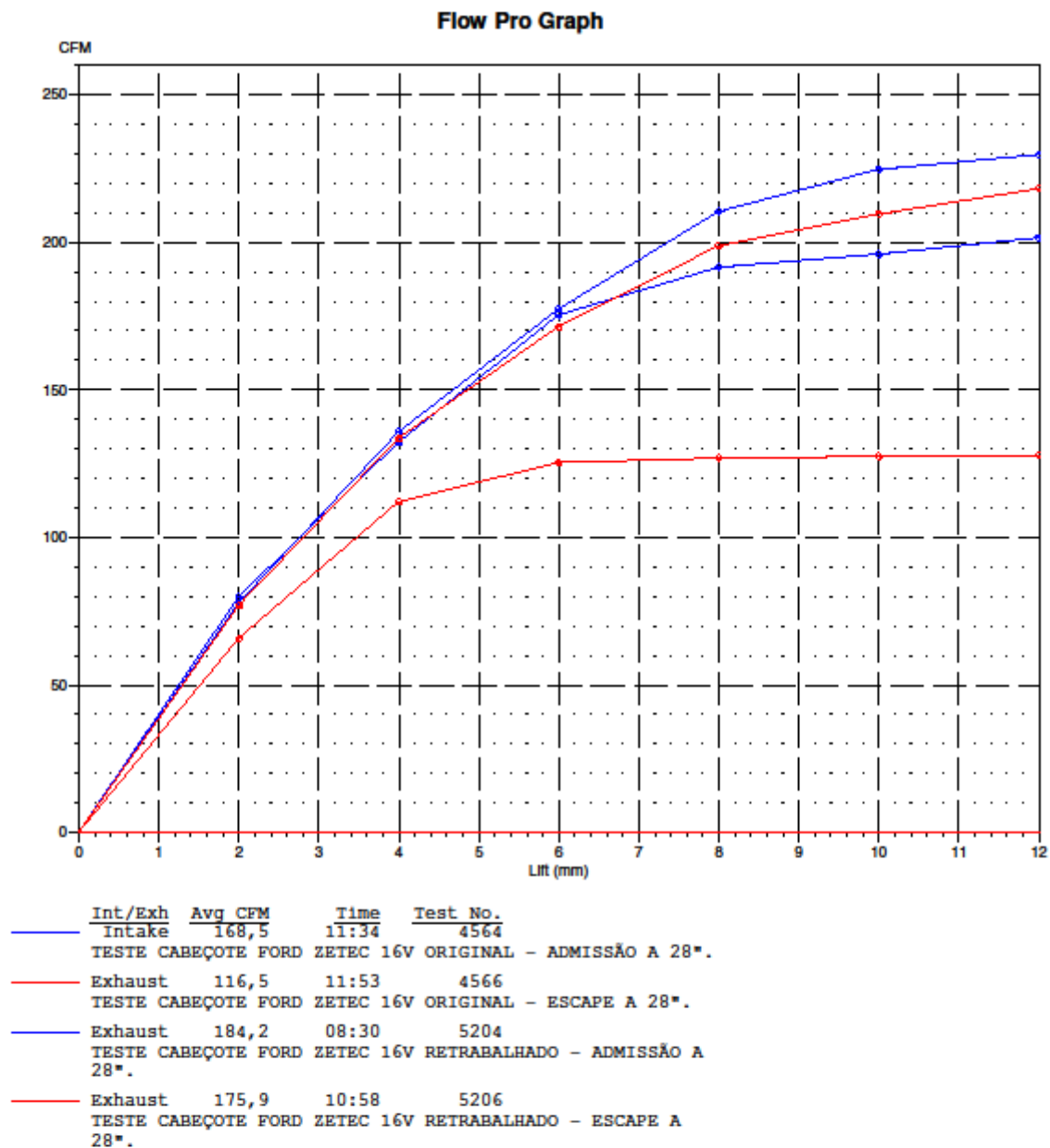
GRAFICO DE FLUXO - CABEÇOTE FORD ZTEC - 16V - COMPARATIVO RETRABALHADO E ORIGINAL A 28"
