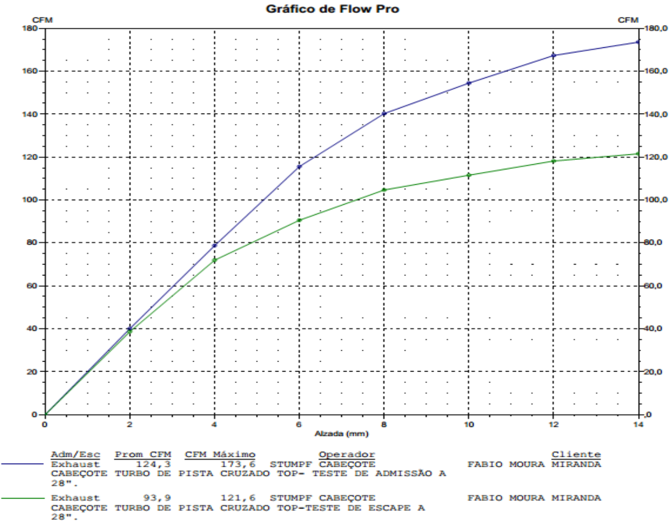
GRAFICO DE FLUXO- CABEÇOTE TURBO DE PISTA CRUZADO TOP- FABIO MOURA MIRANDA
