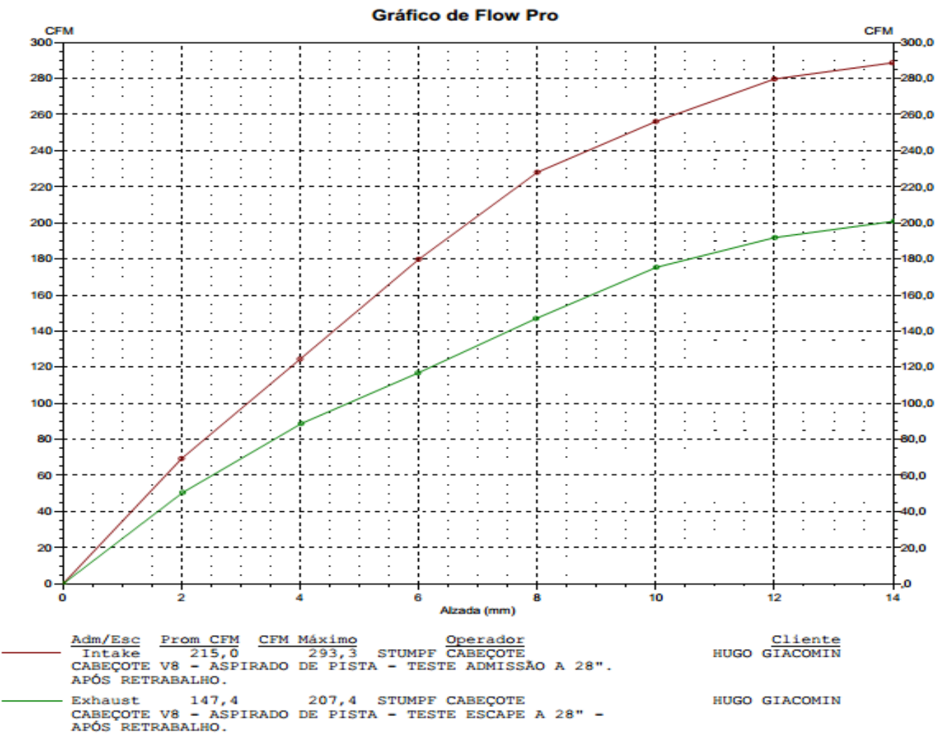
GRAFICO DE FLUXO-CABEÇOTE V8-ASPIRADO DE PISTA-HUGO AUGUSTO GIACOMIN SANTOS
