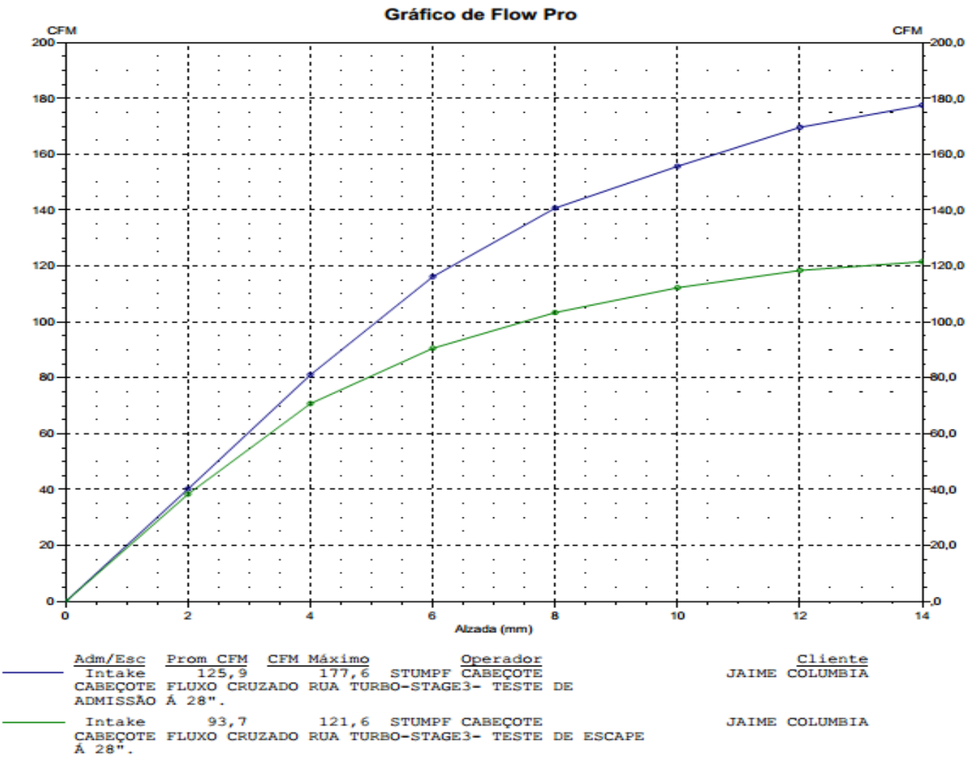
GRAFICO DE FLUXO-CABEÇOTE FLUXO CRUZADO RUA TURBO-STAGE3- JAIME COLUMBIA
