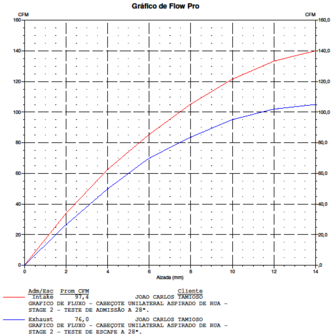
GRAFICO DE FLUXO - CABEÇOTE UNILATERAL ASPIRADO DE RUA - STAGE 2 - JOAO CARLOS TAMIOSO.
