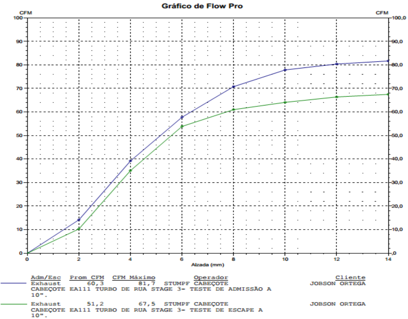
GRAFICO DE FLUXO-CABEÇOTE EA111 TURBO DE RUA STAGE 3-JOBSON ORTEGA
