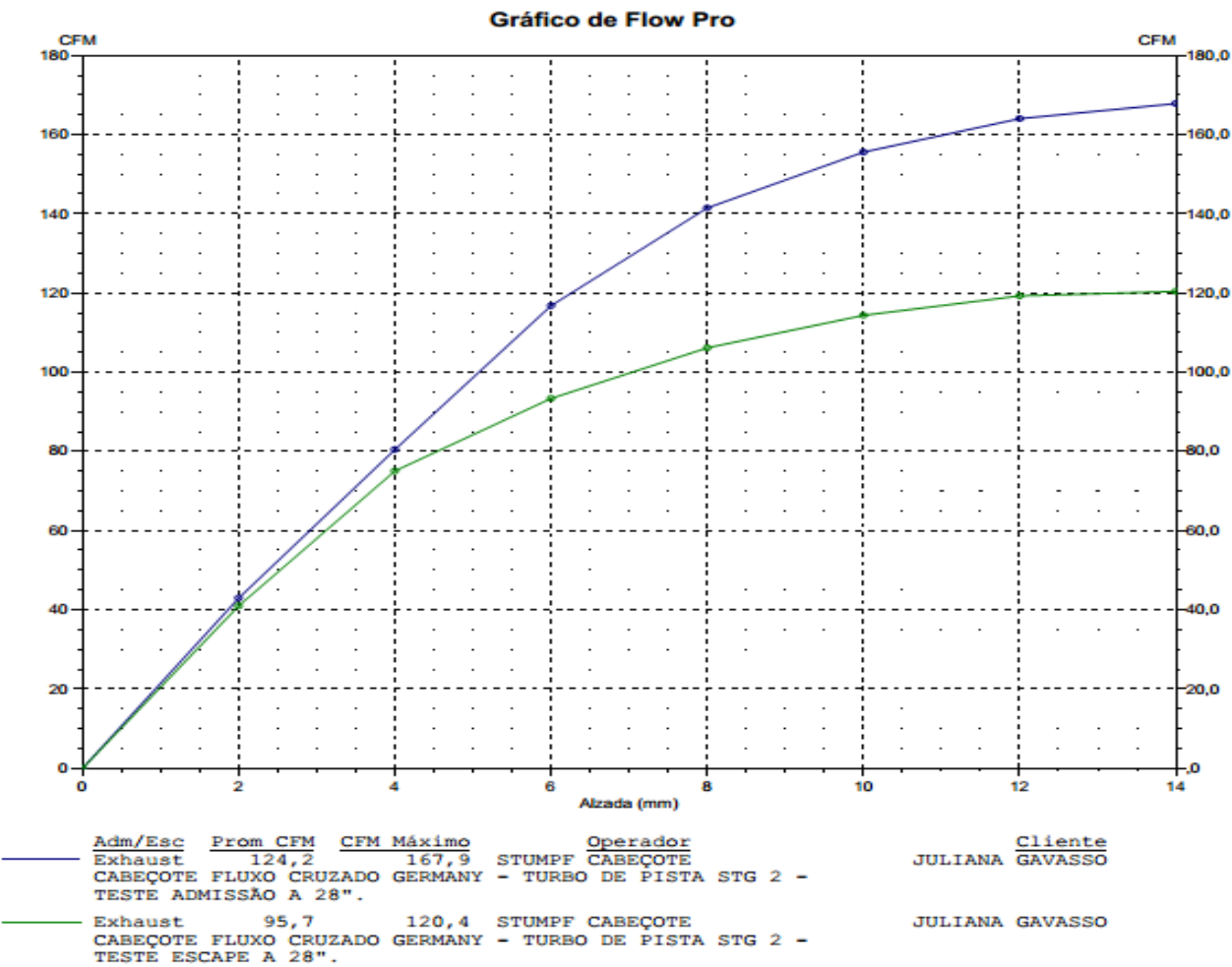
GRAFICO DE FLUXO - CABEÇOTE FLUXO CRUZADO TURBO DE PISTA STG 2 - JULIANA GAVASSO.
