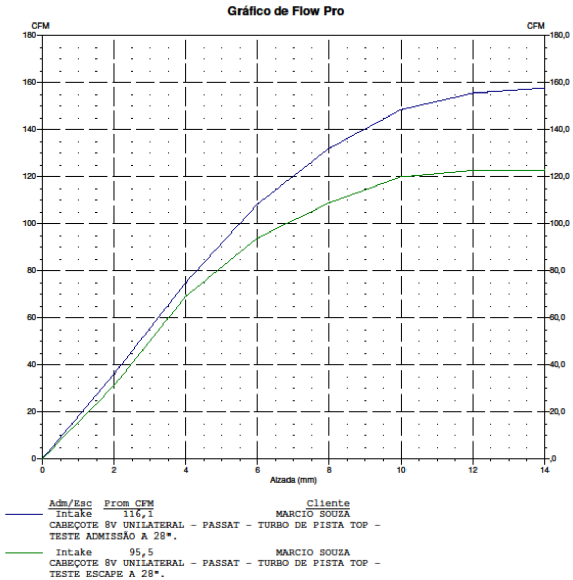
GRAFICO DE FLUXO - CABEÇOTE UNILATERAL - PASSAT - TURBO DE PISTA TOP - MARCIO SOUZA.
