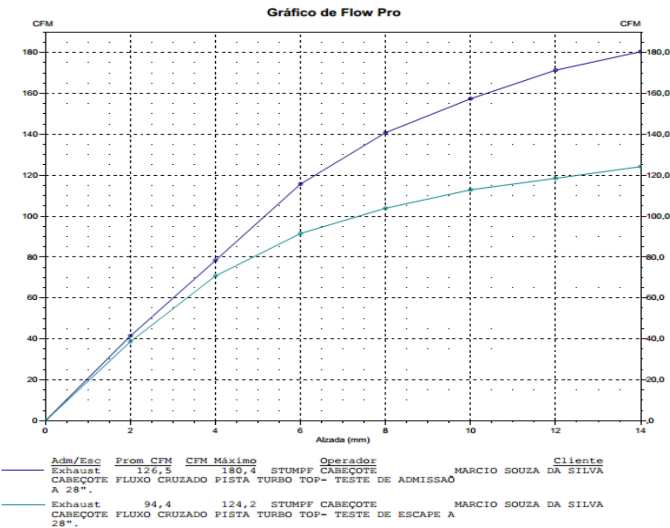
GRAFICO DE FLUXO- CABEÇOTE FLUXO CRUZADO PISTA TURBO TOP- MARCIO SOUZA DA SILVA
