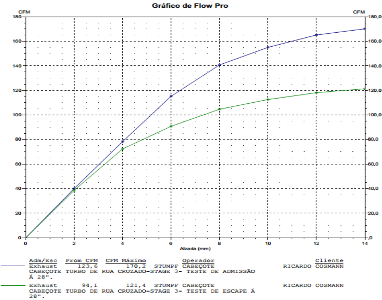
GRAFICO DE FLUXO-CABEÇOTE TURBO DE RUA CRUZADO-STAGE 3- RICARDO COSMANN
