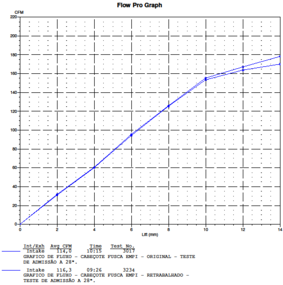
GRAFICO DE FLUXO - CABEÇOTE FUSCA EMPI - RKS PERFORMANCE.
