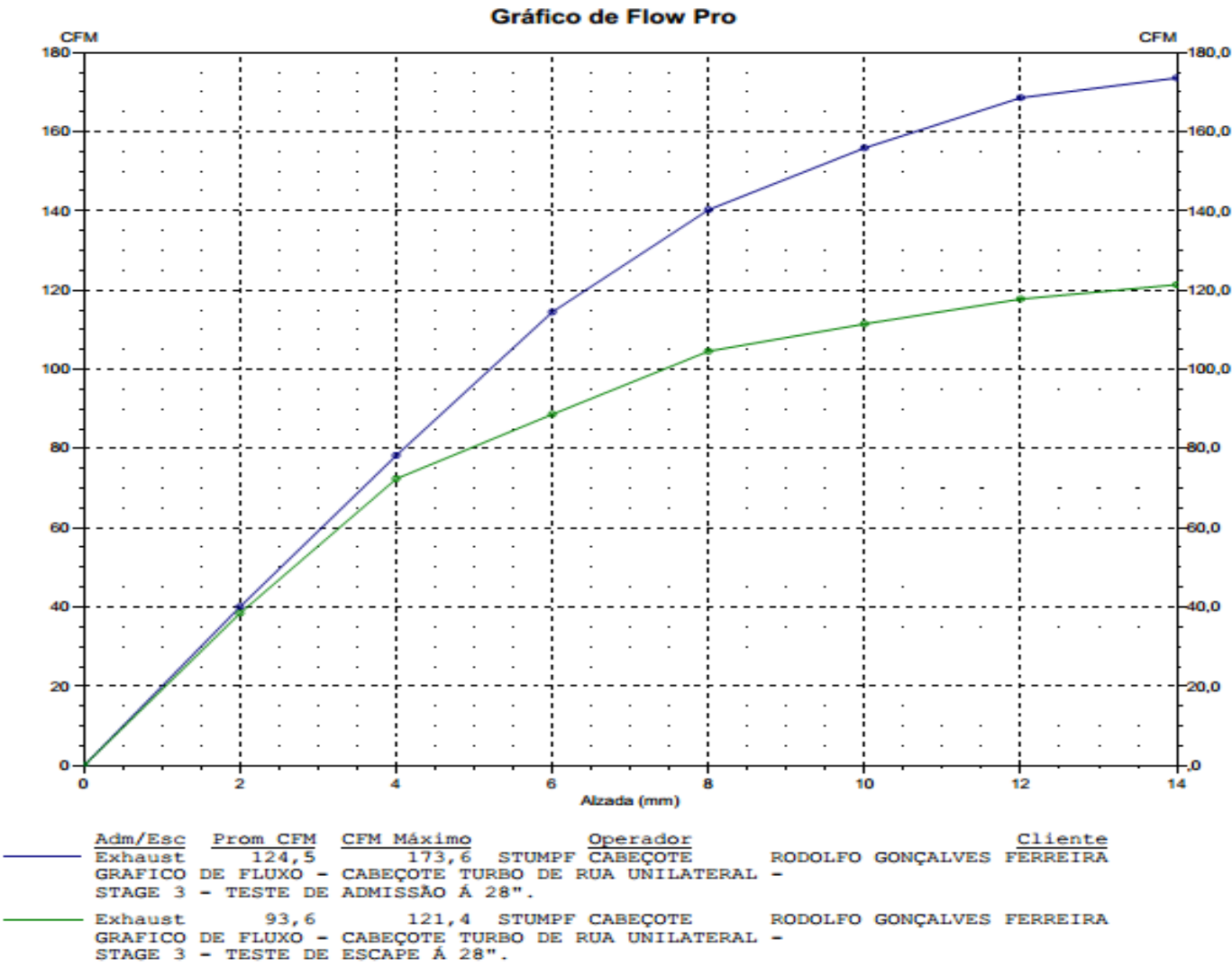
GRAFICO DE FLUXO - CABEÇOTE TURBO DE RUA UNILATERAL - STAGE 3 - TESTE DE ESCAPE À 28".
