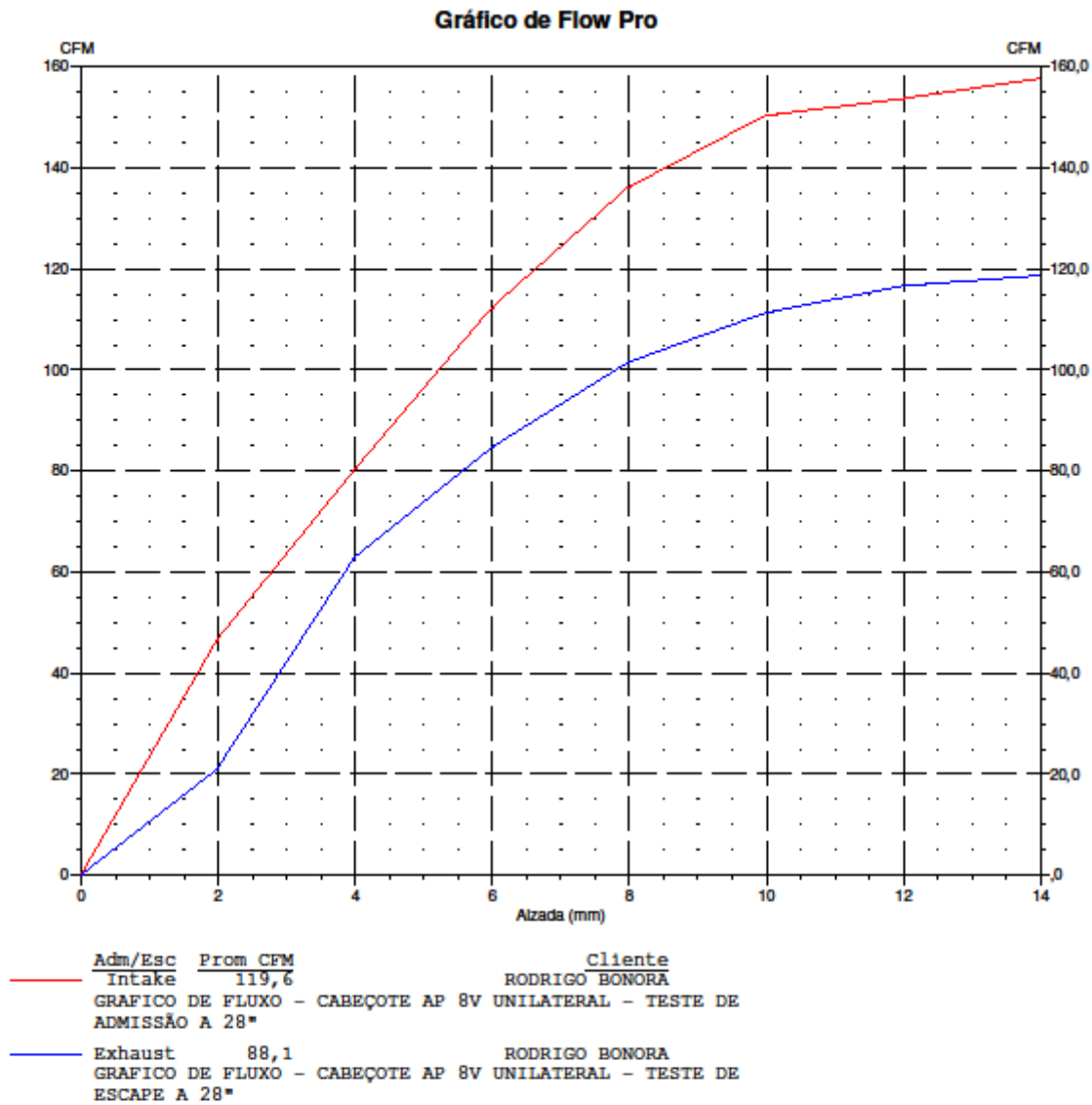
GRAFICO DE FLUXO - CABEÇOTE AP 8V UNILATERAL - RODRIGO BONORA.
