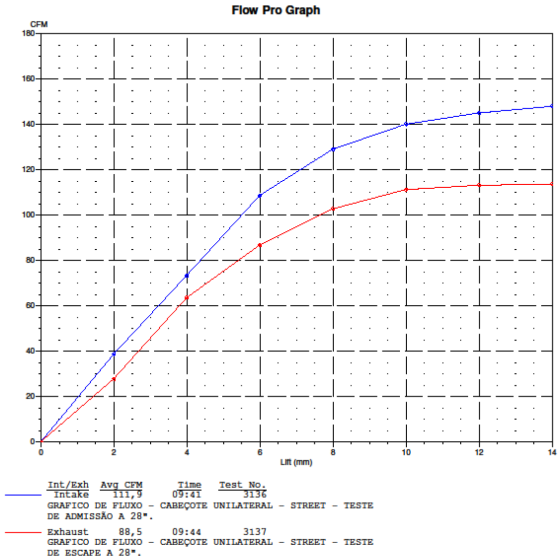
GRAFICO DE FLUXO - CABEÇOTE UNILATERAL - STREET - RONALDO HENRIQUE.
