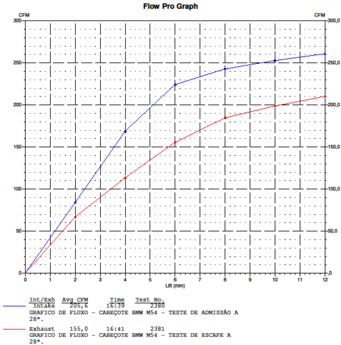
GRAFICO DE FLUXO - CABEÇOTE BMW M54 - SILVIO ALBERTO.
