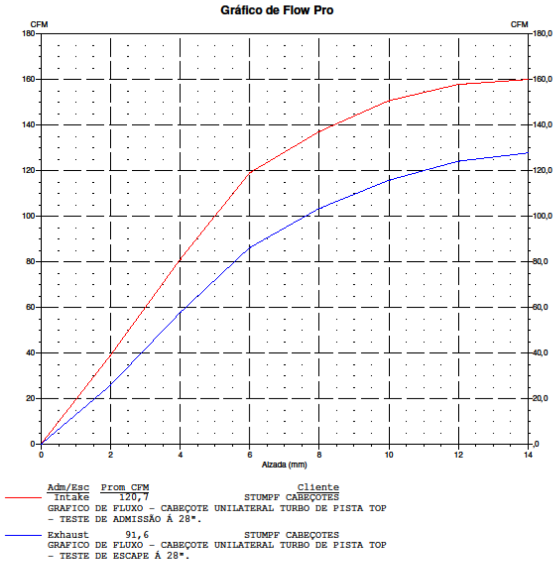
GRAFICO DE FLUXO - CABEÇOTE UNILATERAL TURBO DE PISTA TOP - STUMPF CABEÇOTES.
