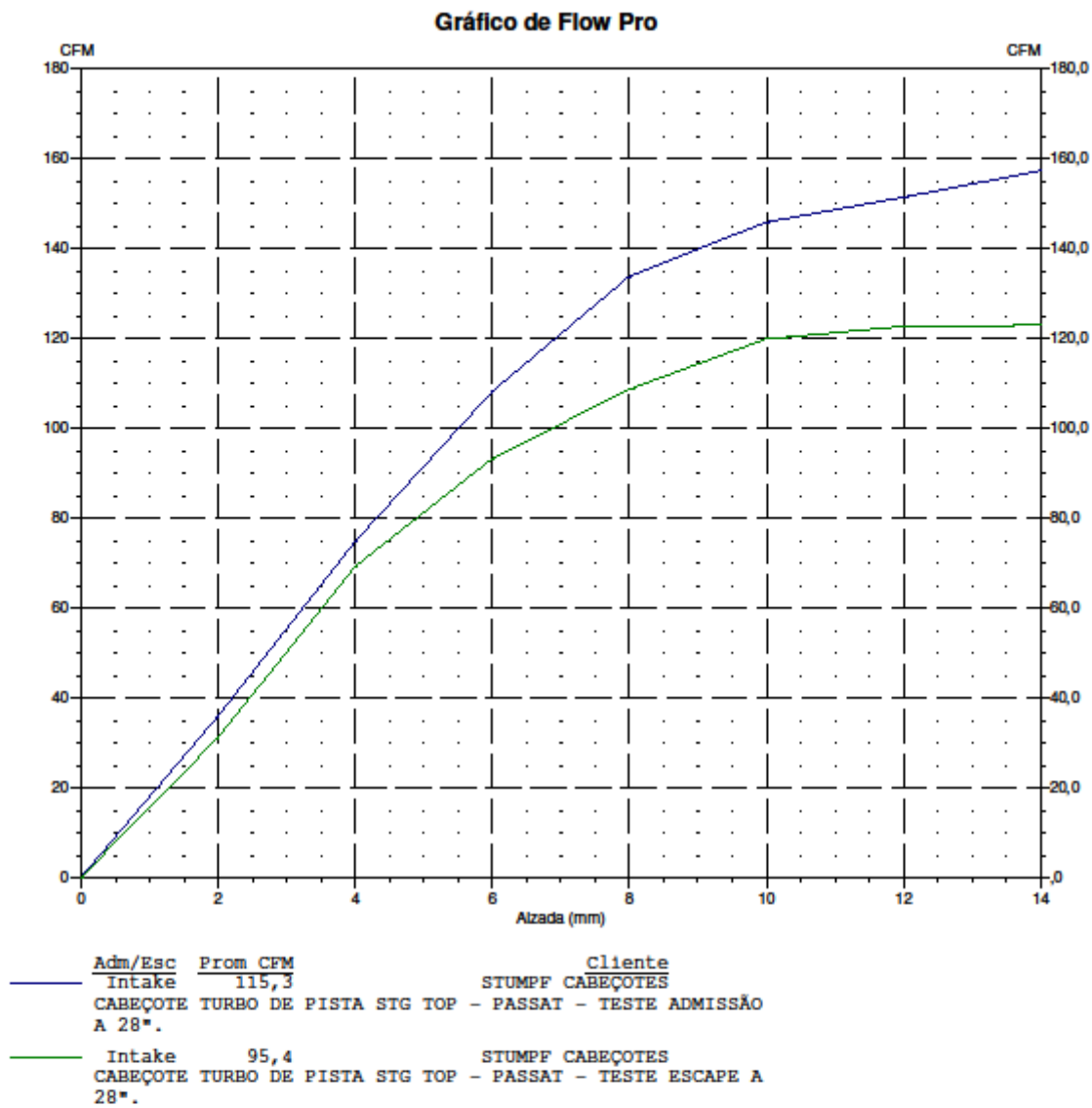
GRAFICO DE FLUXO - CABEÇOTE UNILATERAL PASSAT - TURBO DE PISTA STG TOP.
