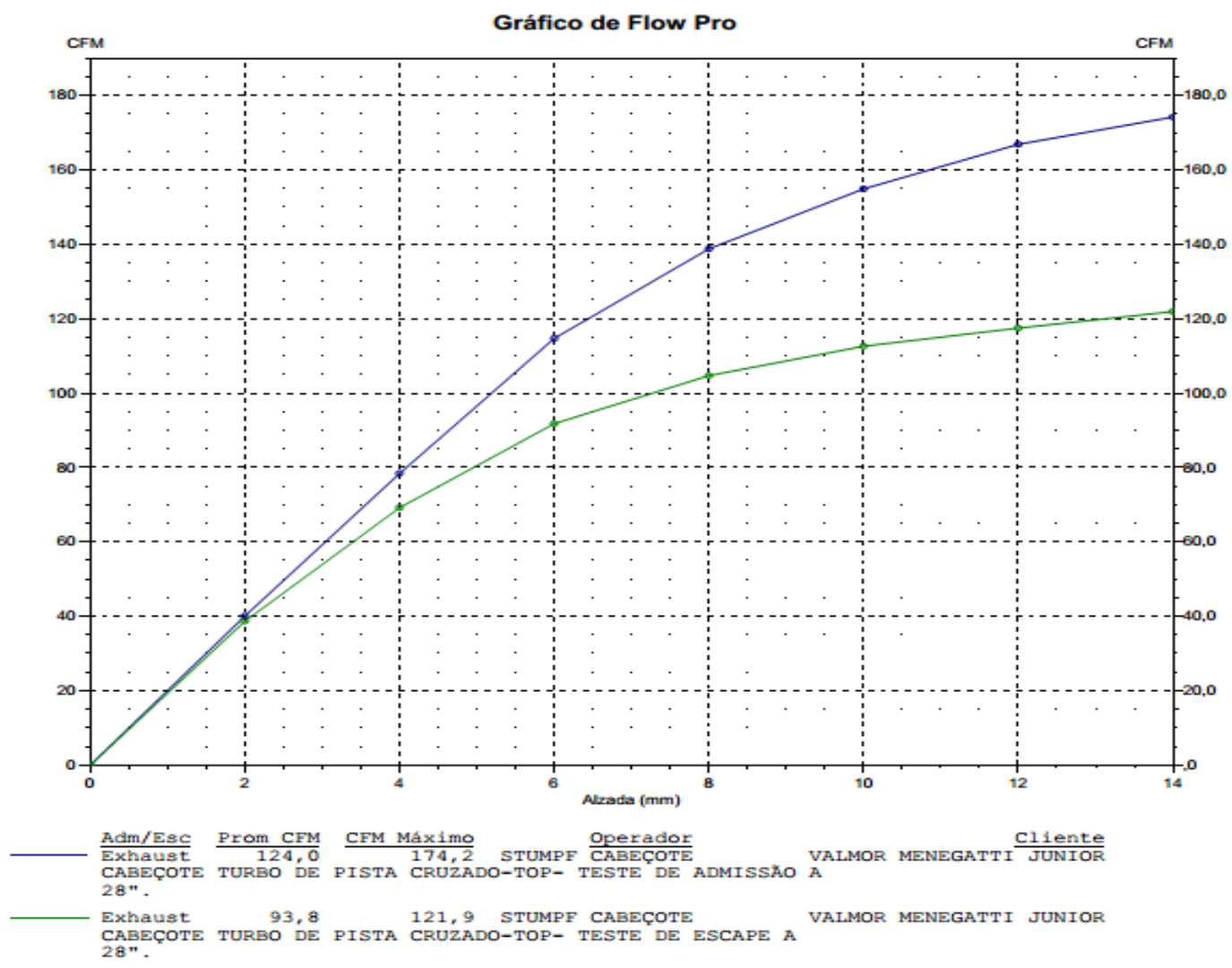
GRAFICO DE FLUXO- CABEÇOTE TURBO DE PISTA CRUZADO-TOP- VALMOR MENEGATTI JUNIOR
