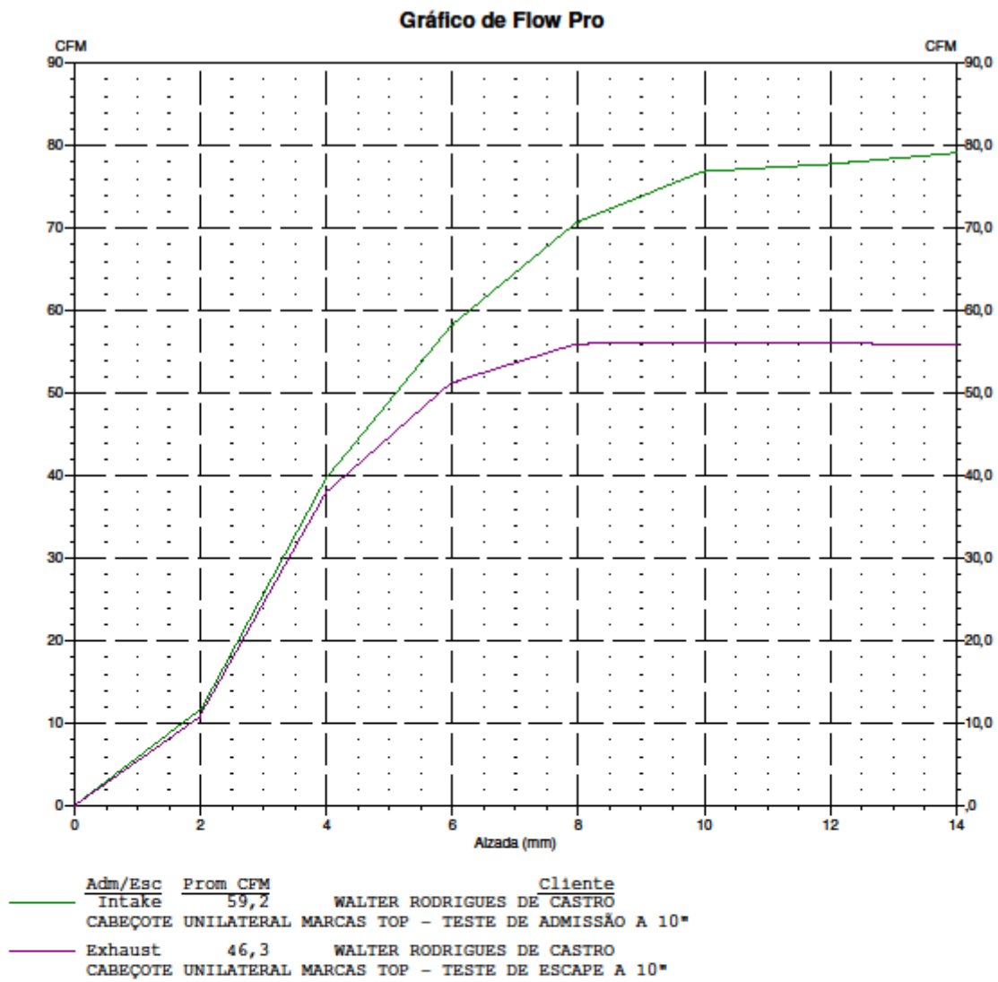
GRAFICO DE FLUXO - CABEÇOTE UNILATERAL MARCAS TOP - WALTER RODRIGUES DE CASTRO JUNIOR.
