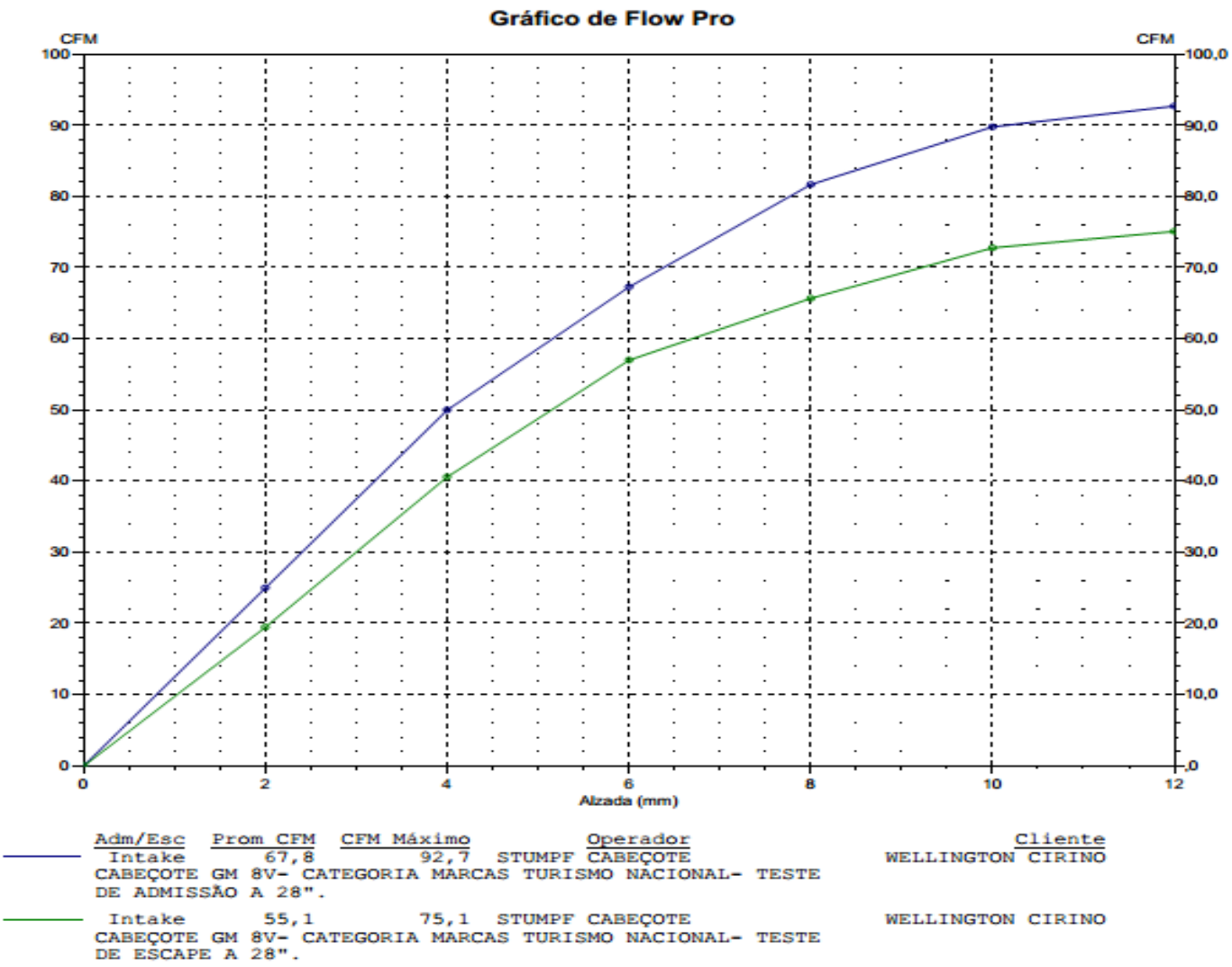
GRAFICO DE FLUXO-CABEÇOTE GM 8V- CATEGORIA MARCAS TURISMO NACIONAL- WELLINGTON CIRINO
